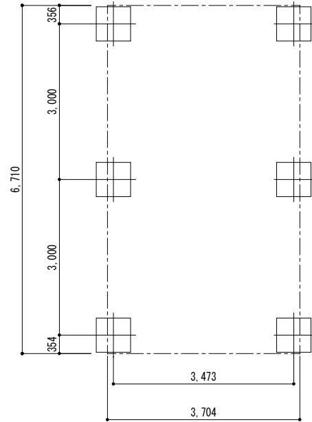
■ 基礎配置図
